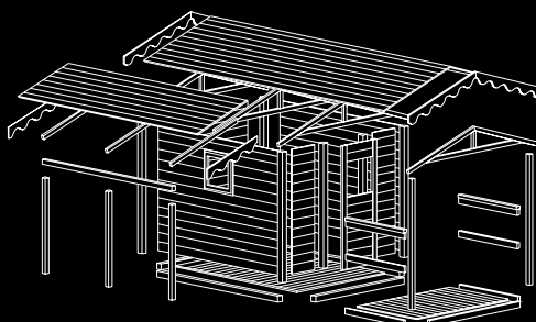
Esploso casetta con tettoia e veranda
