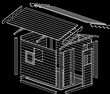
Esploso casetta
