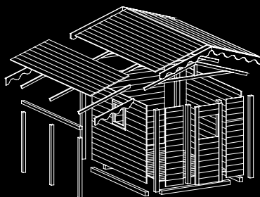
Esploso casetta con tettoia
