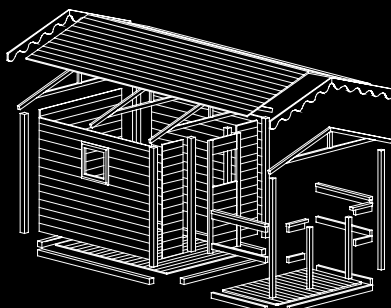
Esploso casetta con veranda
